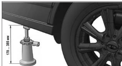
Рис. 83. Замена колеса
